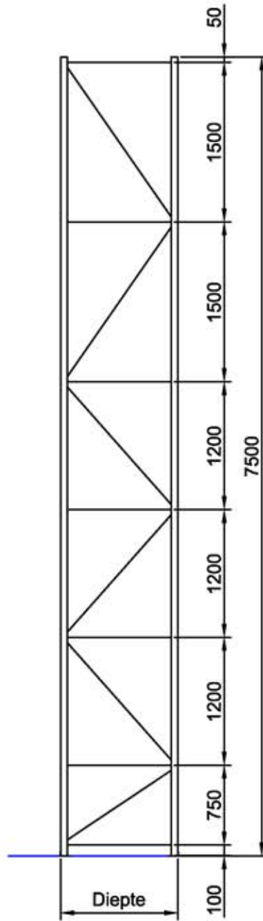
Juk type SKJL
